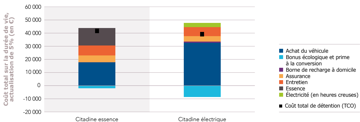
Figure 23. Comparaison des coûts totaux de détention sur la durée de vie entre un véhicule essence et électrique (citadine de catégorie A, basé sur une comparaison entre Renault Clio 5 zen essence et Renault Zoe life 41 kWh)
